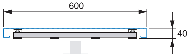
Brzdová deska v příčném řezu
