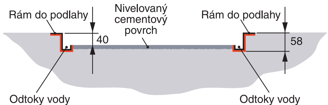
Řez A-B
