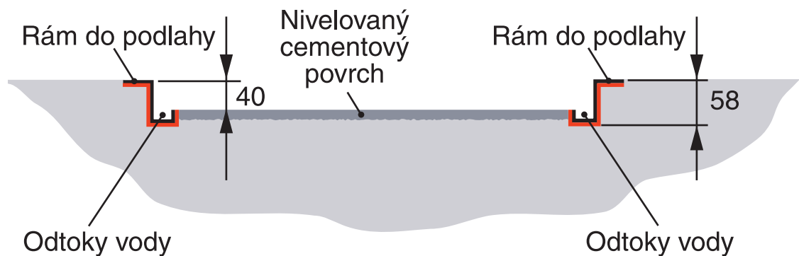
Řez A-B
